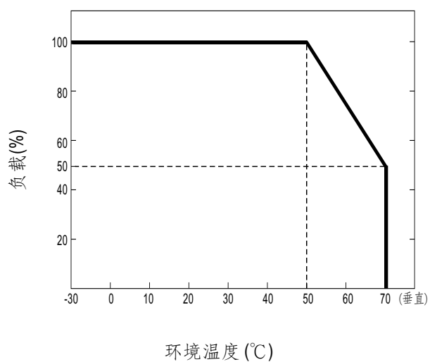
■ 减额曲线
